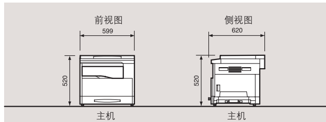
外形尺寸 (单位: mm) (162)
